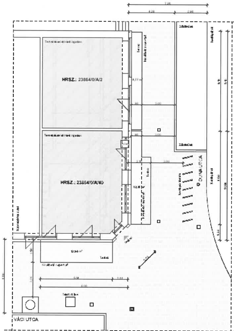
Helyszínrajz M 1:100
