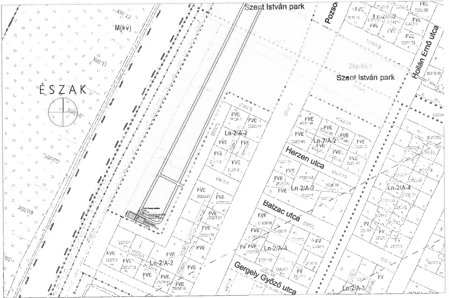
HELYSZÍNERAJZ m=1:1000
