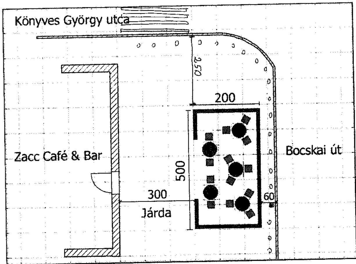
2. kép: Alaprajz (mértékegység - cm)
