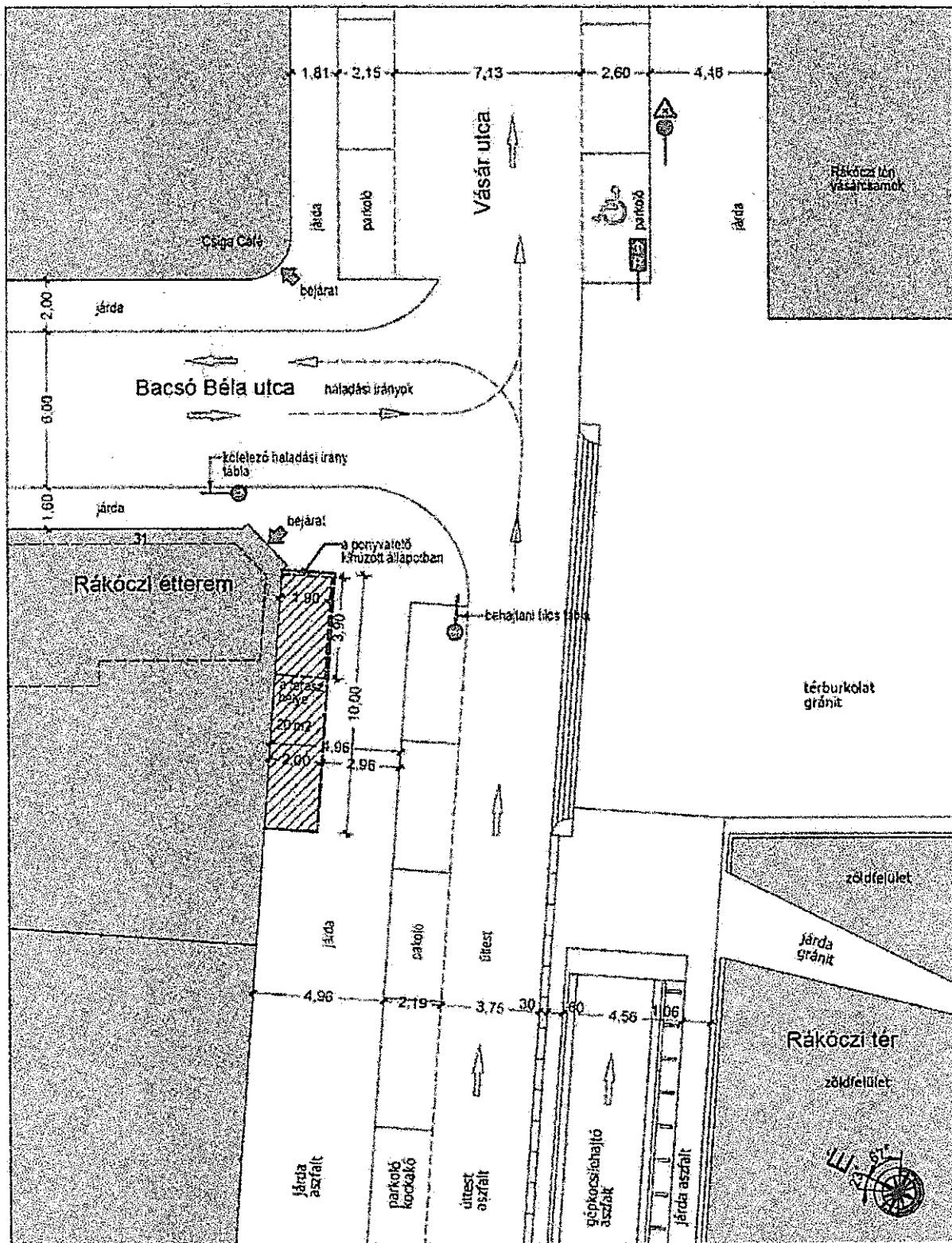
VENDÉGLÁTÓ TERASZ HELYSZÍNRAJZA m=1:200 RÁKÓCZI ÉTTEREM 1083 Budapest, Rákóczi tér 9. Bacsó Béla u. 31. 2020
