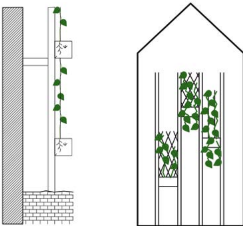
72–73. ábra Homlokzattól független állványrendszerrel, támszerkezetre futtatott kúszónövényvel kialakított zöldhomlokzat (jellegábrák) (Pataky–Csibi)
